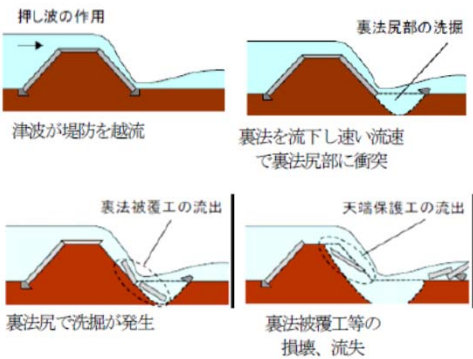
堤防等の破壊のメカニズム
