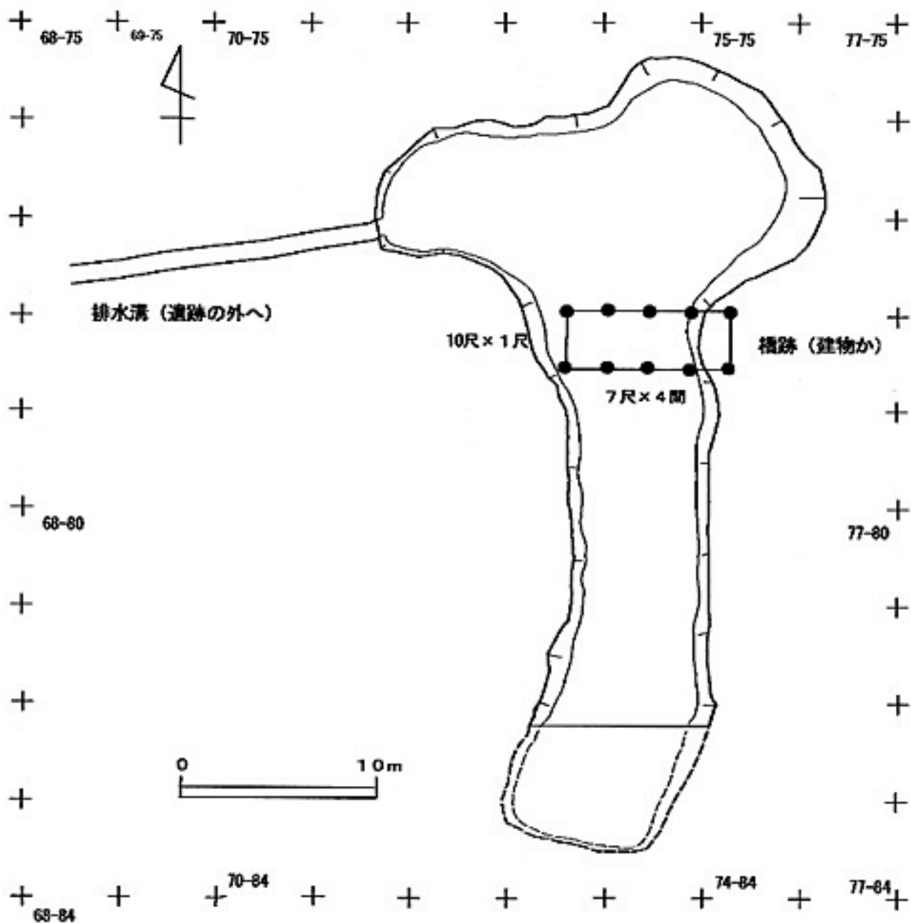
古い段階の池跡平面図
